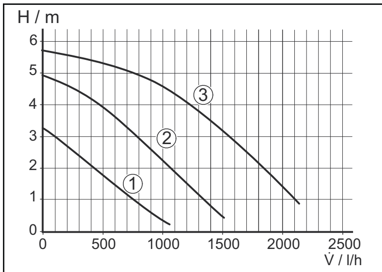
Характеристическая кривая насоса котлов U072 / U072 K
